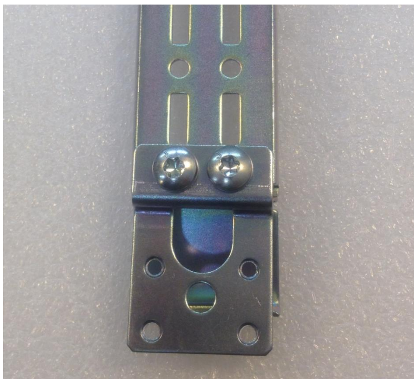
Рис.3.2.8-1 Присоединение удлинителя к шине внутреннего монтажа
